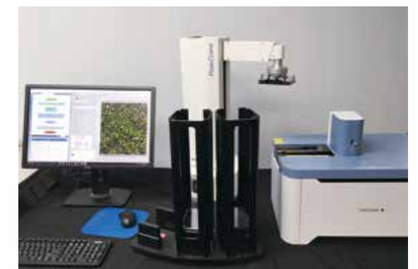
CQ1とスタッカシステムの連携例 構成機器: スタッカ、ロボットハンドラ
