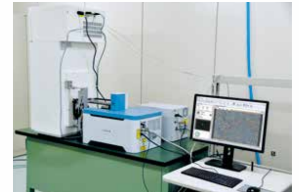
CQ1とインキュベータシステムの連携例 構成機器: インキュベータ、バーコードリーダ、ロボットハンドラ
