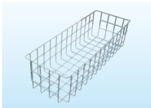
血液バッグ収納バスケット 小型:W162.5×D266×H123mm 標準価格 4,000円 (税抜) 大型:W162.5×D466×H123mm 標準価格 4,700円 (税抜)
